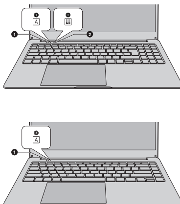
Figura 4-1 Indicatori della tastiera
