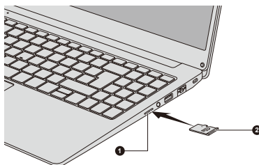
Figura 4-4 Inserimento del supporto di memoria
