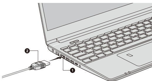
Figura 4-9 Collegamento della porta di uscita HDMI™
