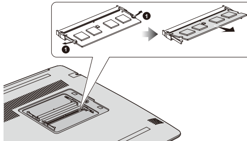
Figura 4-6 Estrazione del modulo di memoria
