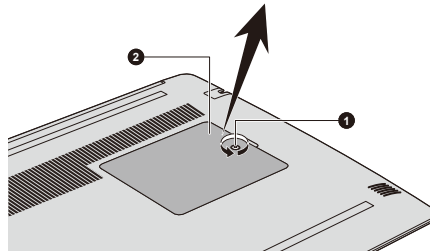
Figura 4-3 Rimozione del coperchio del modulo di memoria
