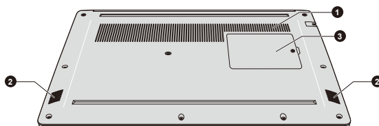
Figura 3-4 Lato inferiore del computer
