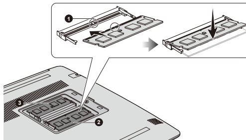
Figura 4-4 Inserimento del modulo di memoria
