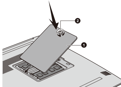
Figura 4-5 Installazione del coperchio del modulo di memoria
