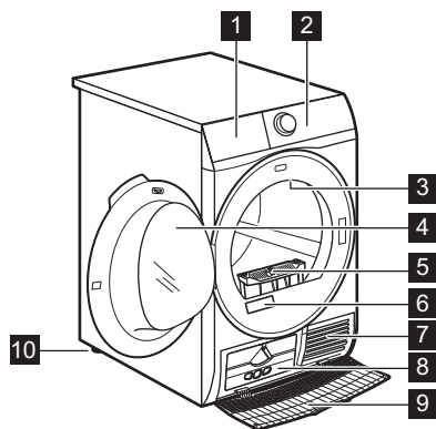
1 Contenitore dell'acqua
