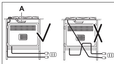
A. Condotta rigida in rame o tubo flessibile in acciaio inox
