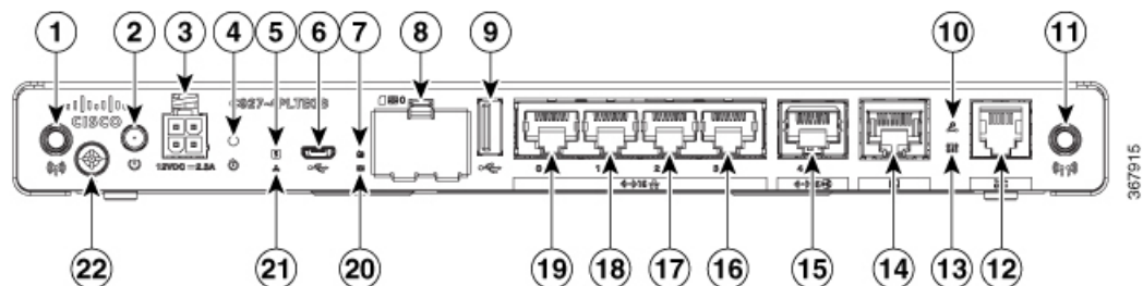
Figura 11: Vista Cisco C927-4PLTEGB - I/O
