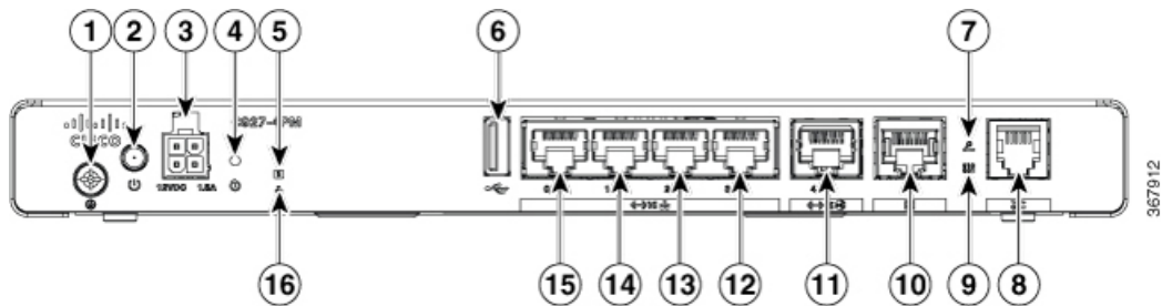
Figura 10: Vista Cisco C927-4PM - I/O
