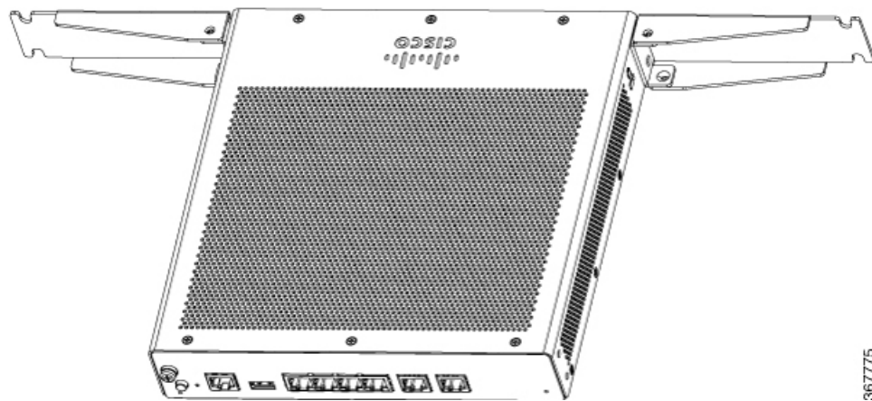
Figura 21: Router con staffa fissata al pannello anteriore
