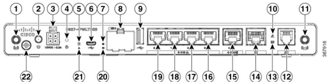
Figura 12: Vista Cisco C927-4PMLTEGB - I/O
