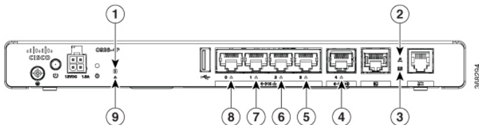
Figura 16: Indicatori LED su SKU DSL - lato I/O
