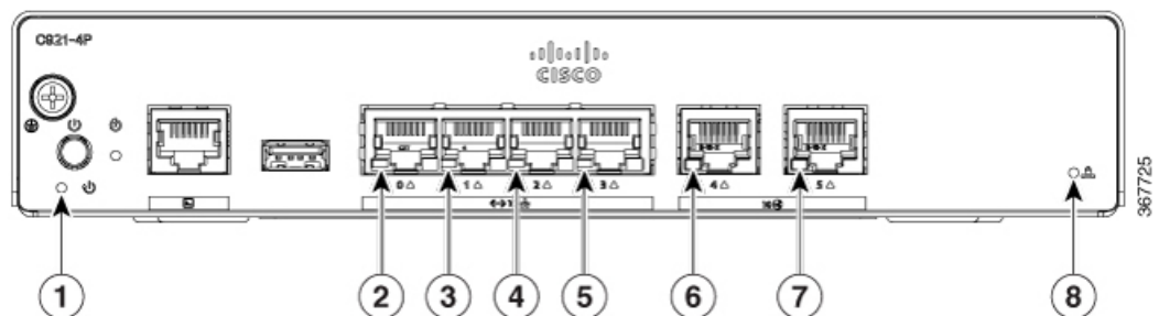
Figura 15: Indicatori LED su SKU Ethernet - lato I/O
