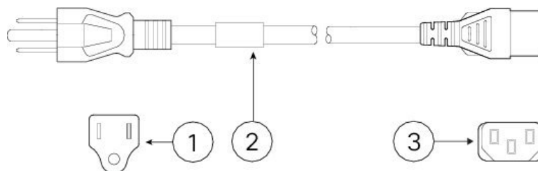
Figura 14: Giappone (CAB-JPN-3PIN)
