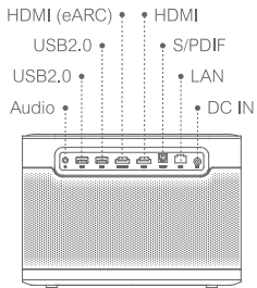
Zadní pohled
