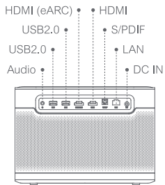
背面視
