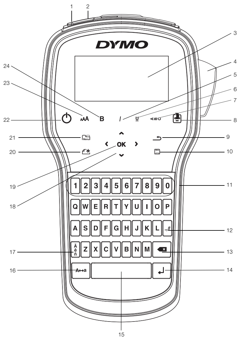
Afbeelding 1 Labelmaker LabelManager 280
