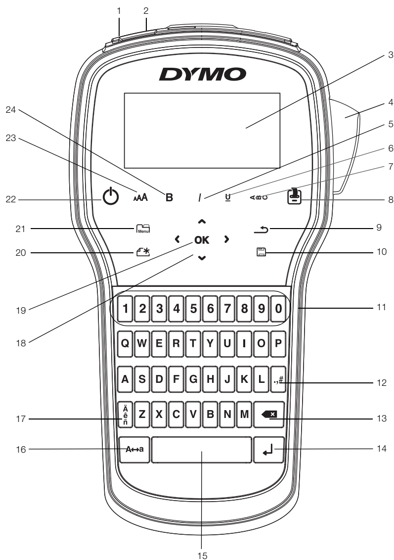
1. ábra LabelManager 280 feliratozógép
