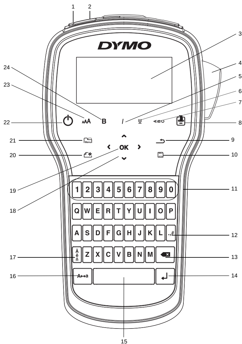
Figura 1 Etiquetadora LabelManager 280
