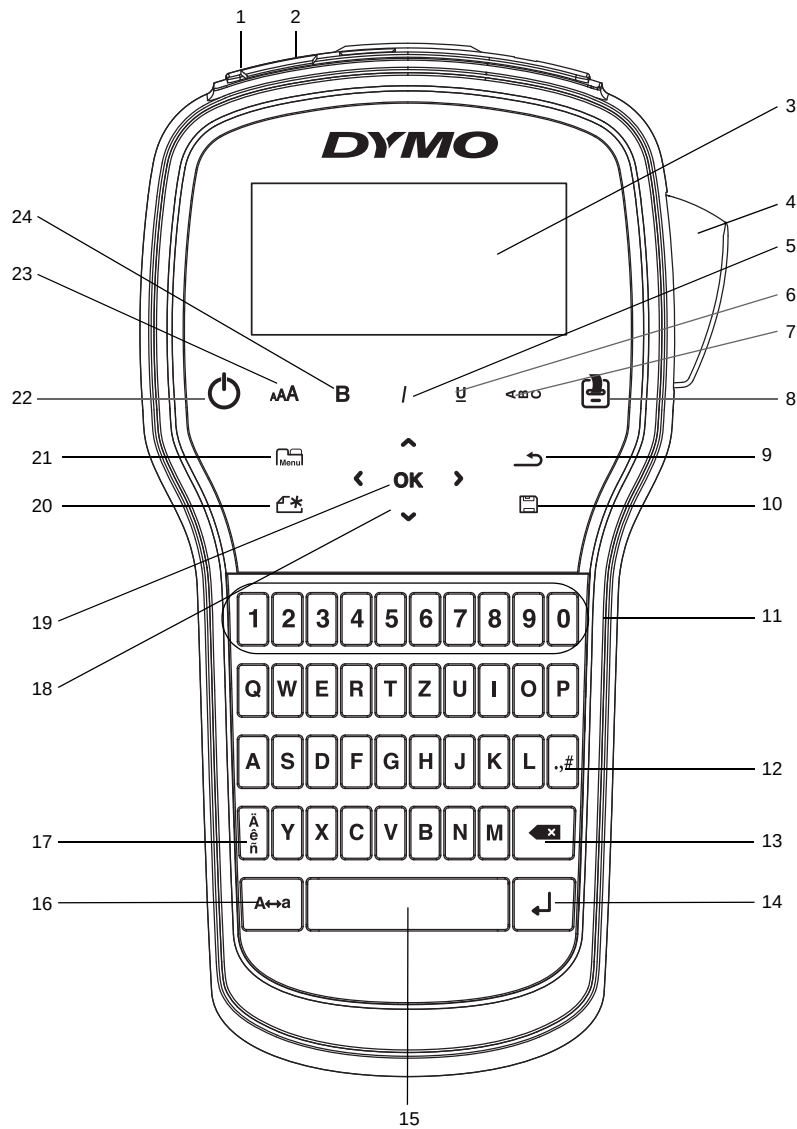
Abbildung 1 LabelManager 280 Etikettendrucker
