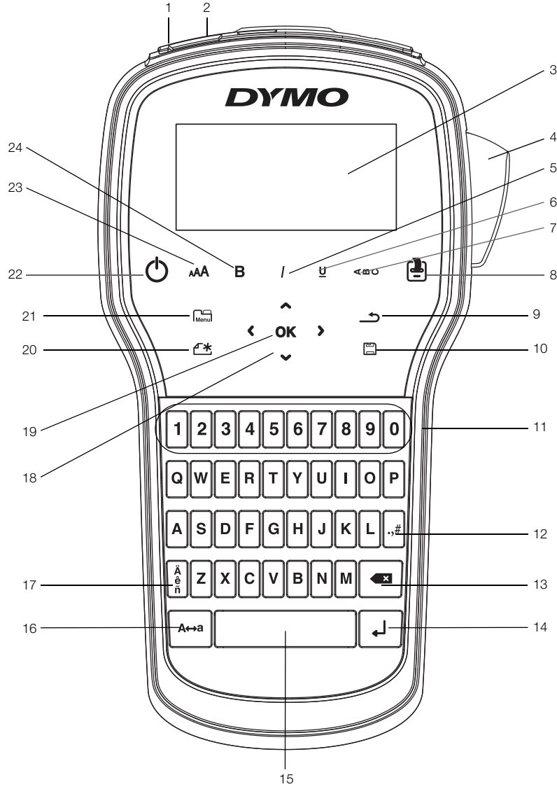
Şekil 1 LabelManager 280 Etiketleme Makinesi
