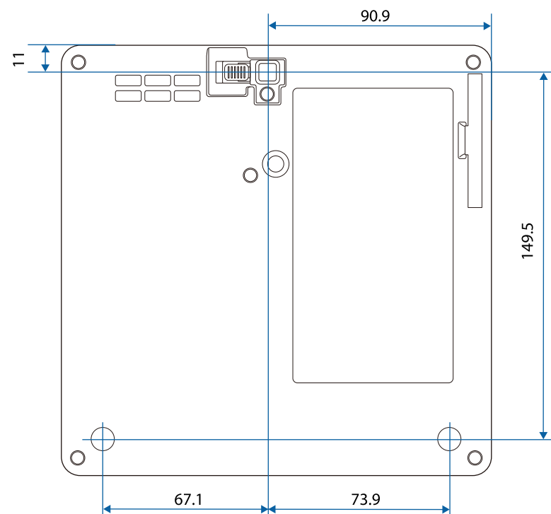
2 Distanza dal centro dell'obiettivo al punto di fissaggio della staffa di sospensione
