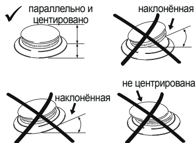
Рис. 9: положение пламерассекателей
