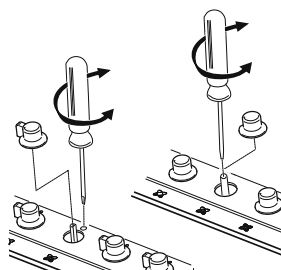
Fig. 8 : réglage du minimum
