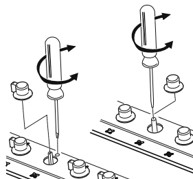
Obr. 8: regulace minimálního plamene
