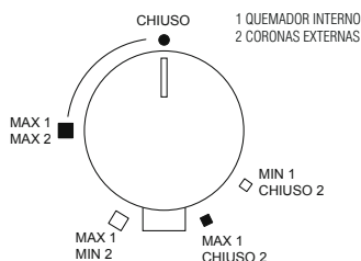
Fig. 12: manilla quemador dual (S4000) / doble corona
