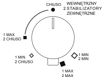
Rys. 13: pokrętło palnika dual (GIOTTO/VULCANO)
