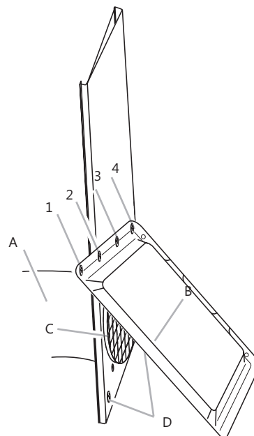
A. Выхлопной переходник для окна B. Защита от дождя C. Вытяжная воздухоораспределительная решётка D. Болты вставляются в неиспользуемые отверстия в комплекте ползунка для окна
