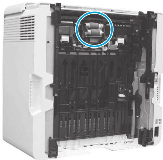
Figura 9-17 Pulizia dei rulli
