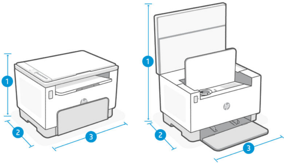
Figure A-1 Dimensioni della stampante (modelli dn/dw/w/USB)
