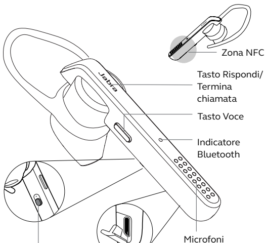
Interruttore On/Off
