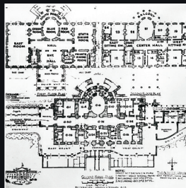
I disegni delle modifiche del 1948 di Lorenzo Winslow. Museo della Casa Bianca
