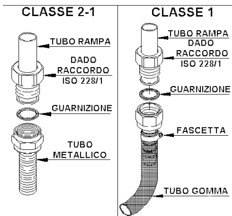
SCHEMA COLLEGAMENTO DEL TUBO FLESSIBILE TRA BOMBOLA E CUCINA CON PORTAGOMMA
