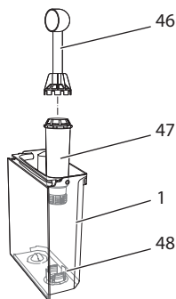
Afb. 25: Waterfilter in-/uitschakelen
