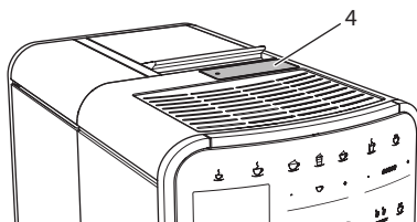
Abb. 10: Pulverschacht
