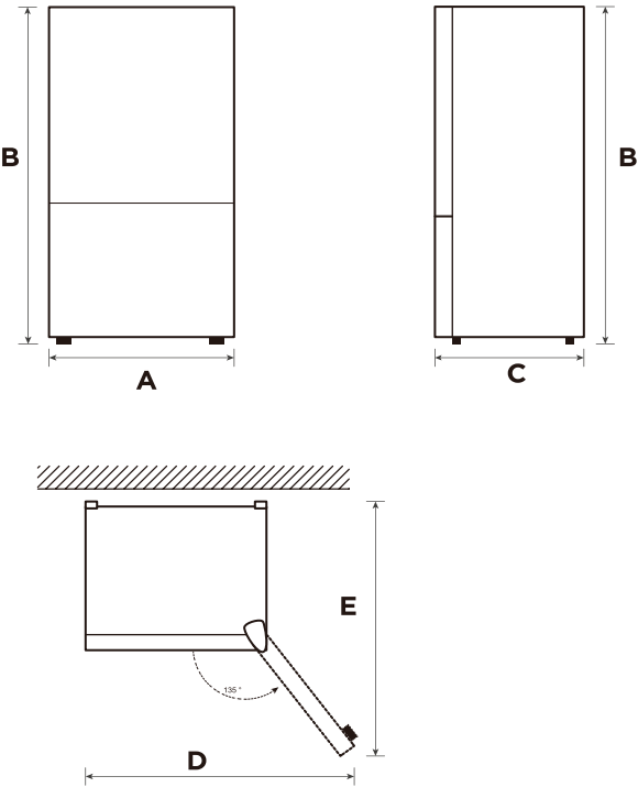
Диаграма на пространствените изисквания (при отворена и при затворена врата)
