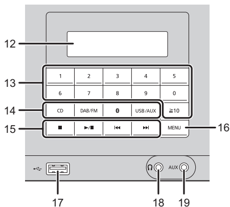
Čelní pohled
