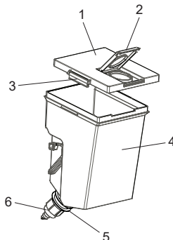
Conjunto del depósito de agua
