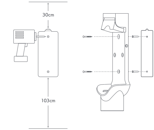
設置推奨高度：シール下部と床面の間隔が 103cm 以上
