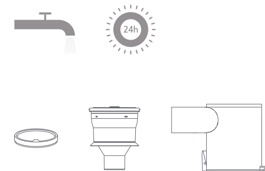
Filtr wstępny Zespół cyklonowy Pojemnik na kurz
