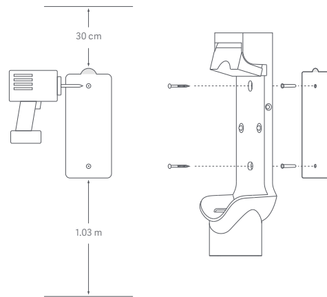
الارتفاع الموصي به: 1.03 متر من الأرض على الأقل
