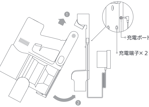
スタンドを利用して充電する場合
