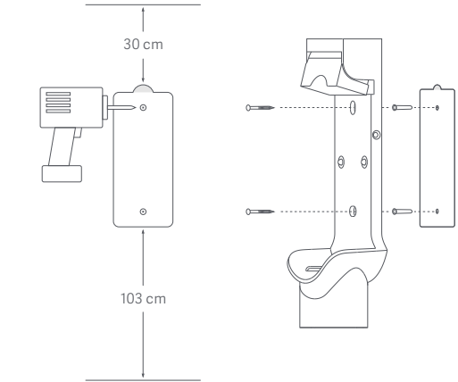
Aanbevolen hoogte: Minstens 1,03 meter vanaf de vloer
