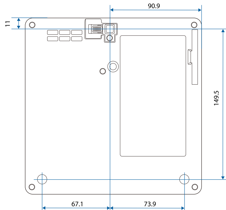
② Distanza dal centro dell'obiettivo al punto di fissaggio della staffa di sospensione
