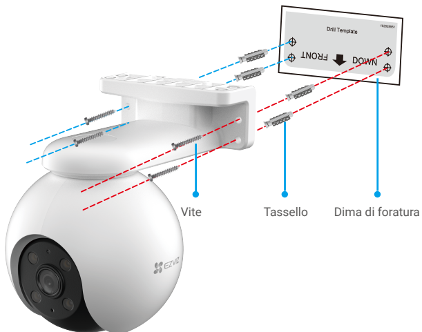
Fig. 2 Montaggio a parete
