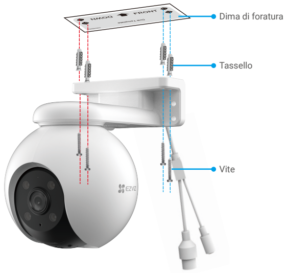
Fig. 1 Montaggio a soffitto
