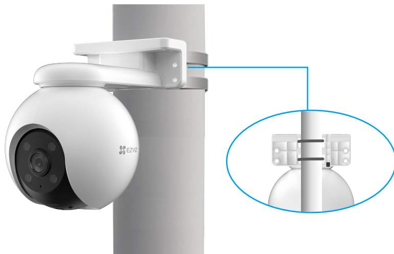
Fig. 3: Montaggio in verticale su palo
