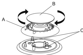
Sl.10: postavljanje plamenika III serije
