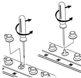
Obr. 8: regulace minimálního plamene
