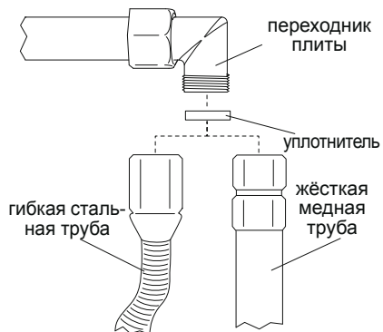
Рис. 6: подключение к сети газового снабжения
