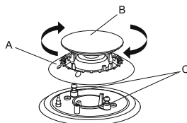
Rys. 10: umieszczenie palnika III serii
