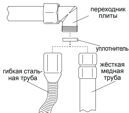
Рис. 6: подключение к сети газового снабжения
