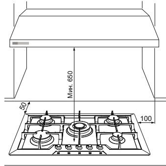
Рис. 3: расстояния плиты
