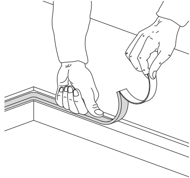
Rys. 5: umieszczanie uszczelnienia
