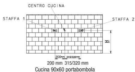
Cucina 90x60 portabombola
