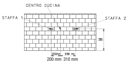
Cucina 80x50 portabombola
