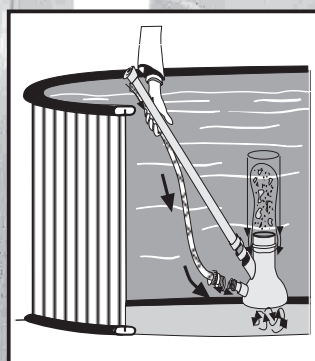
VENTURY STYLE TIPO VENTURY APIRATEUR VENTURI BODEMMEUGER VENTURY LIMPA-FUNDOS VENTURI BODEMMEUGER VENTURY LIMPA-FUNDOS VENTURI
