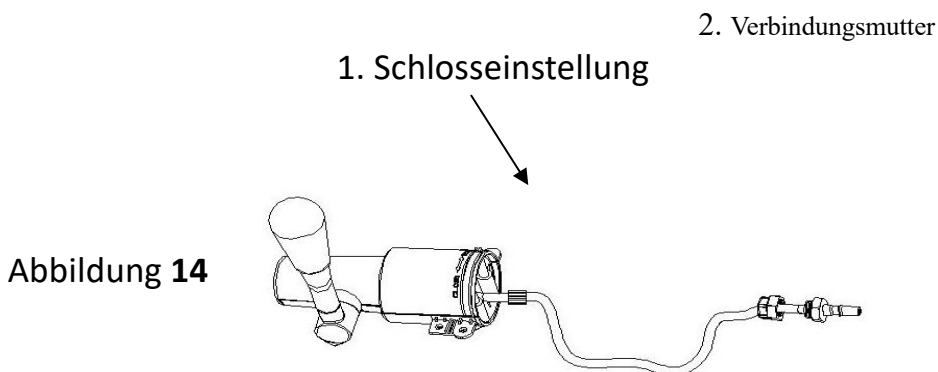
Die Bierleitung
