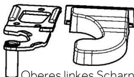
Oberes linkes Scharnier für den Wechsel des Türanschlags Scharnierabdeckung oben links
