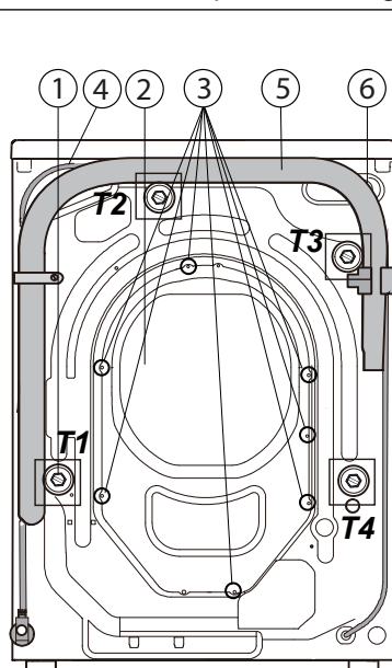
Lato posteriore (Fig. 2-2):
