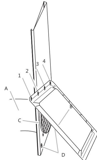
A. Fenster Auspuffadapter B. Regen Abdeckung C. Austrittsgitter D. Bolts in unbenutzten Löcher in Fenster Slider-Kit eingesetzt
