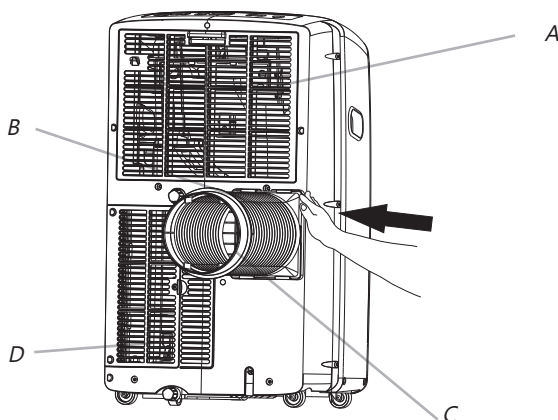
A. Verdampers luchtinlaat B. Dummy koppeling C. Flexibele afvoerslang D. Condensor luchtinlaat
