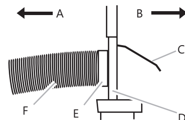
A. Vers le climatiseur B. Extérieur C. Cache antipluie D. Kit coulissant pour fenêtre E. Adaptateur d'évacuation d'air F. Tuyau d'échappement flexible
