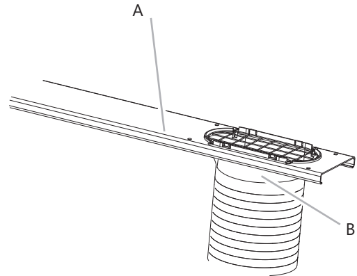
A. Venster schuifregelaar pakket B. Venster uitlaatadapter
