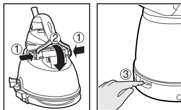
Fig. 4: Ontgrendelen en aanzetten van het striksysteem.
