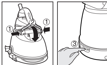
Fig. 4: Sbloccare ed accendere il sistema stirante
