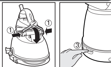
Εικ.4 Ξεκλειδώστε και ανάψτε το σύστημα σιδερώματος
