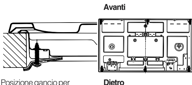
Posizione gancio per top H=40mm
