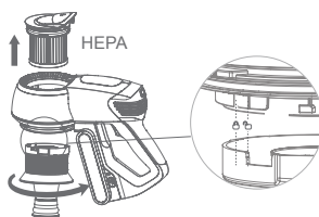
Grade 2-Zyklonkomponenten
