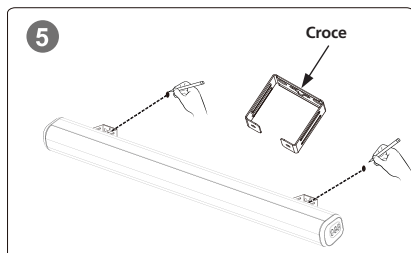
Fase 5 Utilizzare le staffe come modello e segnare i punti di foratura sulla parete. A tal fine, utilizzare la croce nel supporto.
