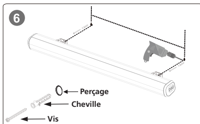
Étape 6. Percez les trous, insérez les chevilles et vissez les vis. Fixez ensuite le support mural par la croix aux vis.
