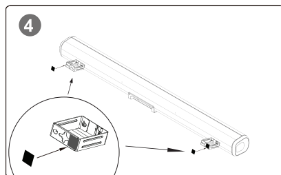
Fase 4 Fissare 2 pezzi di materiale espanso EVA (senza fori) alle due staffe a muro come da illustrazione.
