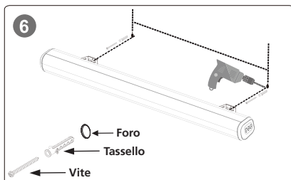
Fase 6 Praticare i fori, inserire i tasselli e avvitare le viti. Quindi fissare la staffa a parete con la croce alle viti.
