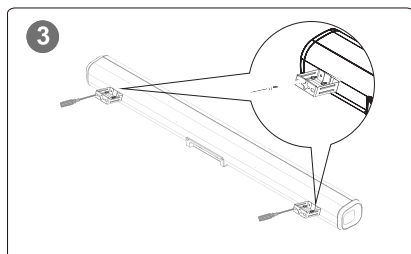
Étape 3. Fixez les 2 supports à la barre de son à l'aide des 4 vis retirées précédemment.
