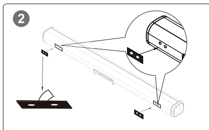
Fase 2 Incollare 2 pezzi di materiale espanso EVA (con fori) su Soundbar e allineare i fori con quelli di Soundbar.
