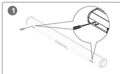
Fase 1 Rimuovere le 4 viti da Soundbar.
