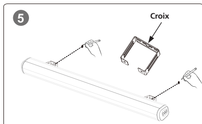
Étape 5. Utilisez les supports comme gabarit et repérez le point à percer sur le mur. Utilisez à cet effet la croix sur le support.
