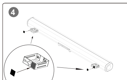
Étape 4. Installez les 2 mousses EVA (sans trous) aux deux supports muraux conformément à la figure.
