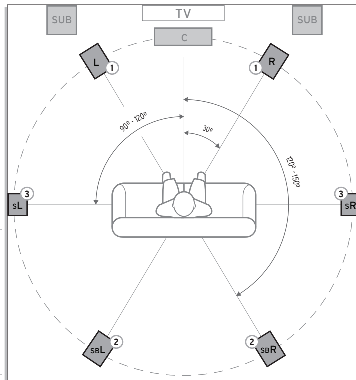
COLLOCAZIONE DEGLI ALTOPARANTI NELL'AREA DI ASCOLTO
