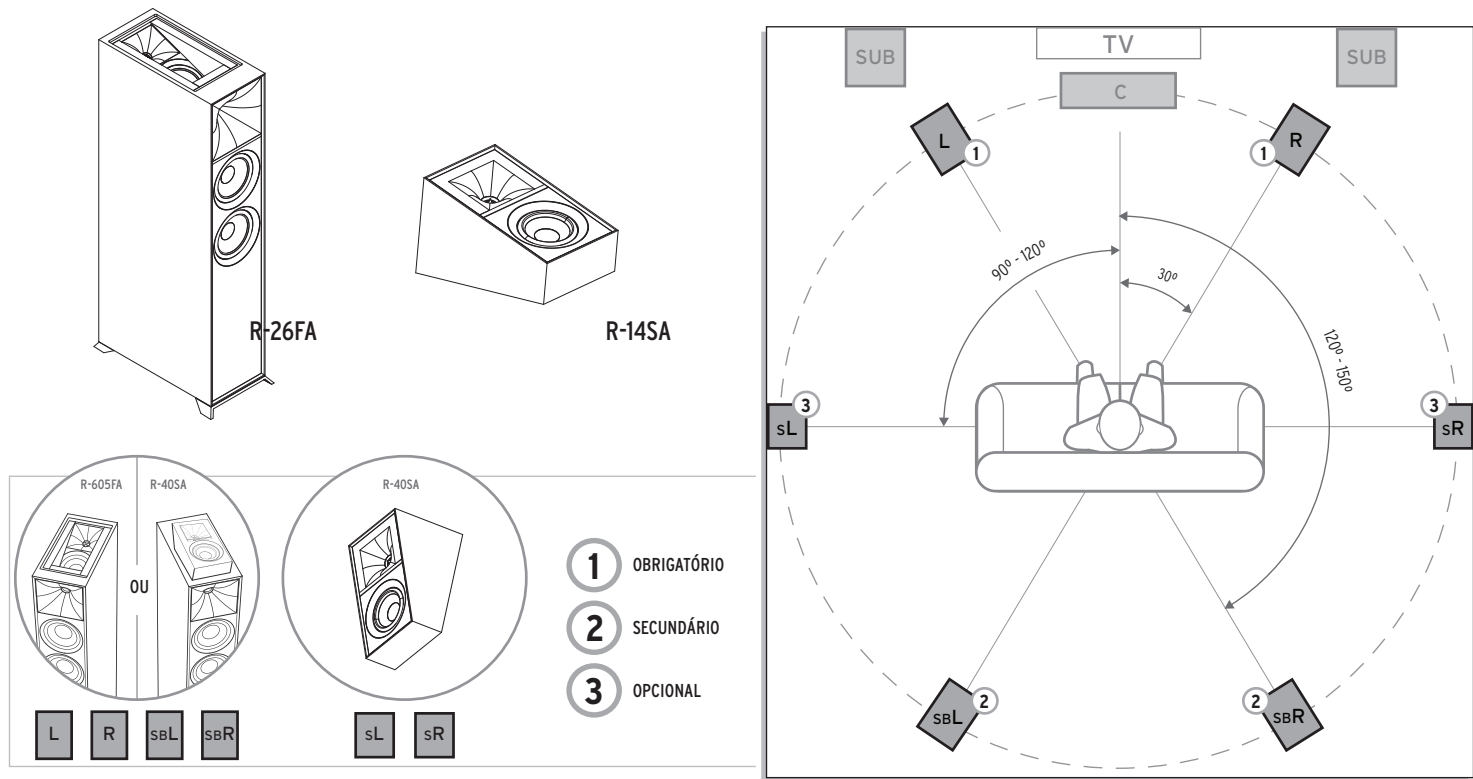
POSICIONAMENTO DAS CAIXAS ACÚSTICAS NO AMBIENTE
