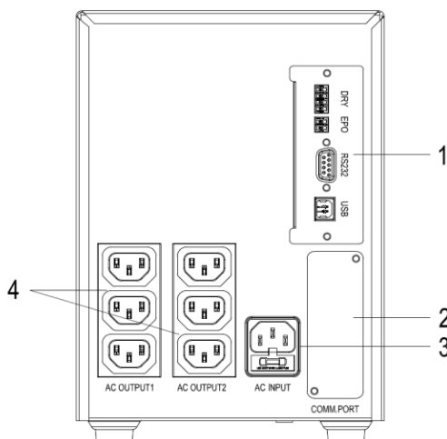
Vue arrière du 750VA
