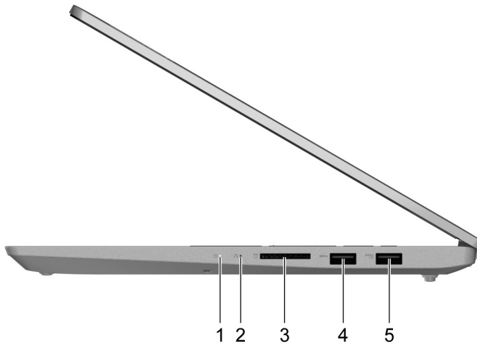
Figura 8. IdeaPad 5 (15", 05) e IdeaPad Slim 5 (15", 05) - vista laterale destra
