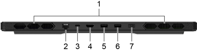
Figura 5. Legion Pro 7 16IRX9H—vista posteriore
