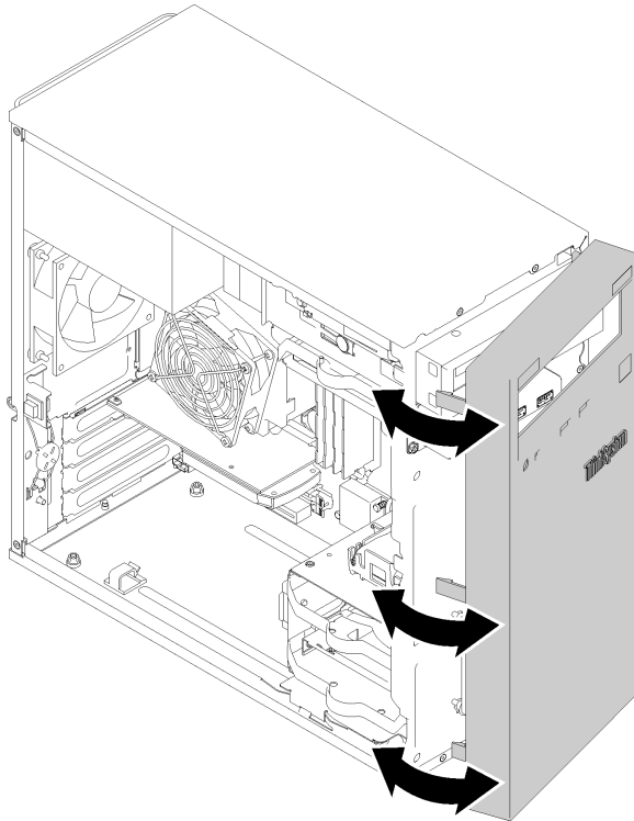
Figura 32. Rimozione della mascherina anteriore
