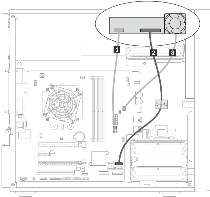
Figura 20. Instradamento dei cavi per l'adattatore del vano dell'unità con unità disco fisso o SSD
