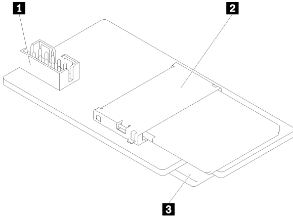
Figura 10. Modulo adattatore per scheda SD doppia
