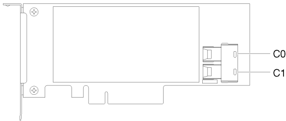
Figura 11. Connettori dell'adattatore RAID SATA/SAS (8i)
