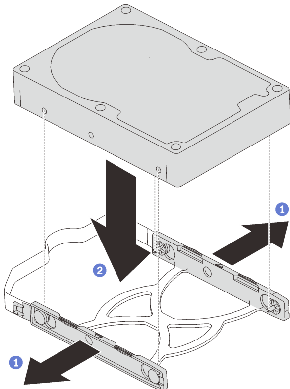
Figura 46. Installazione di un'unità da 3,5" nel supporto
