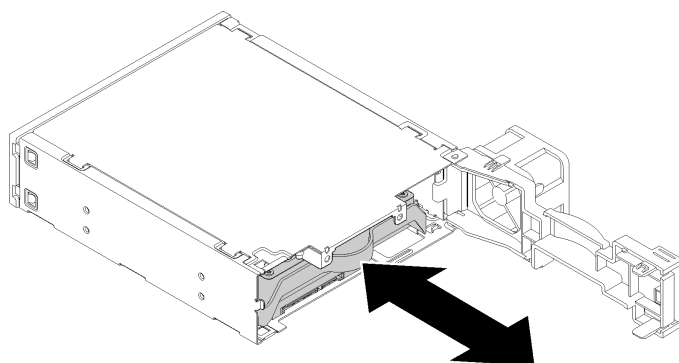
Figura 47. Installazione dell'assieme dell'unità nell'adattatore dell'unità
