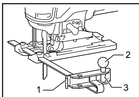
1. Guide de garde 2. Boulon fileté 3. Broche du guide circulaire
